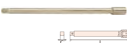
Verlängerung aus Titan Titanium Driver Extension
